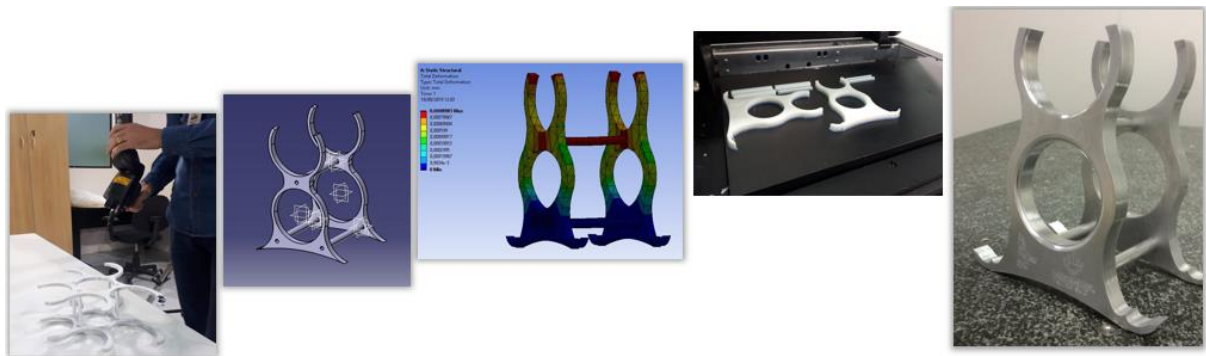
Brinde feito pelo Laboratório para a 6ª RM Vale TI (Engenharia reversa; Desenho 3D; Simulação Estrutural; Impressão 3D e Usinagem).
