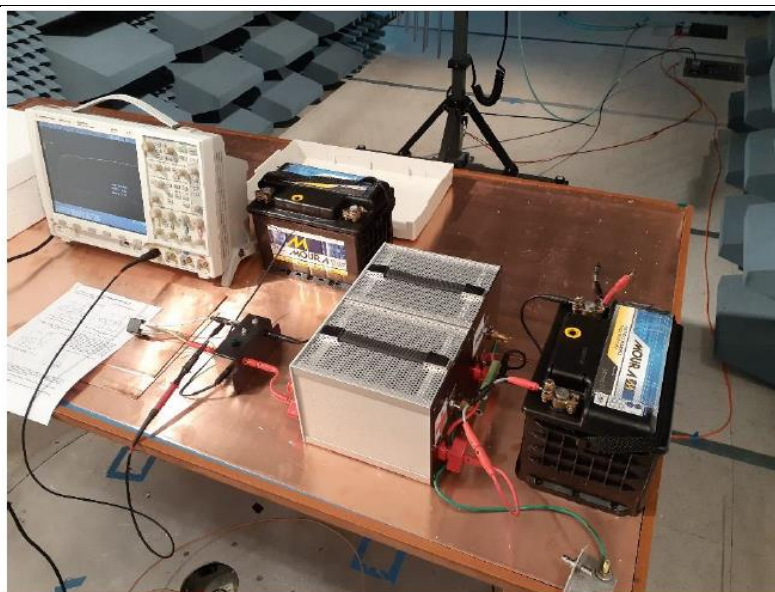
Setup de teste de Emissão Conduzida de Transientes.
