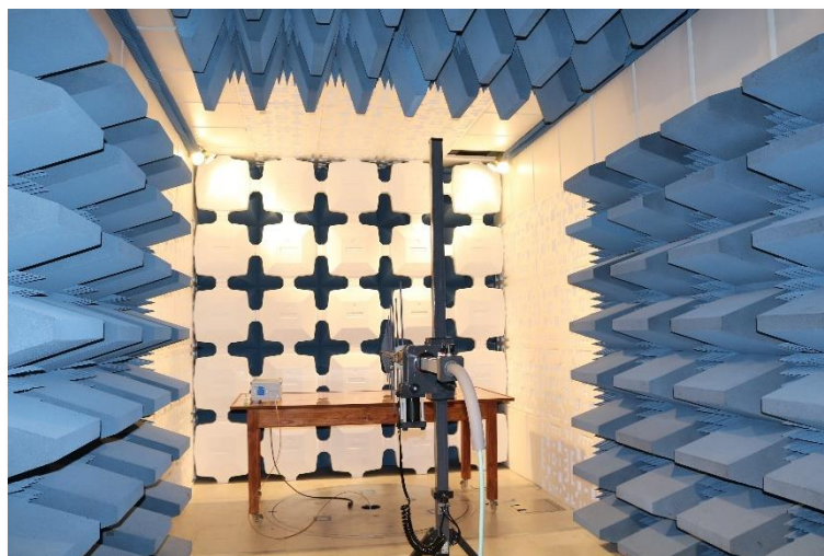
Laboratório de EMI/EMC do PqTec em operação.
