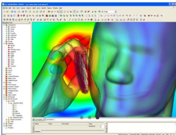
Ilustração do software CST (Imagem do site da Smattech).
